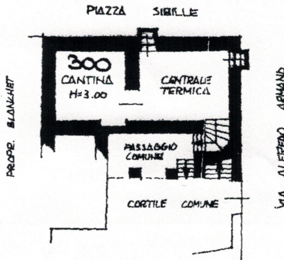
PIANO SOTTERRANEO
